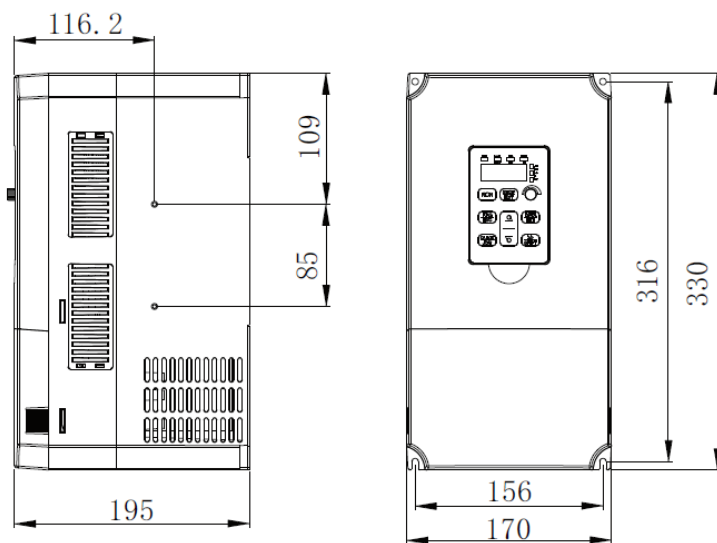
11KW—15KW 结构示意图及尺寸
