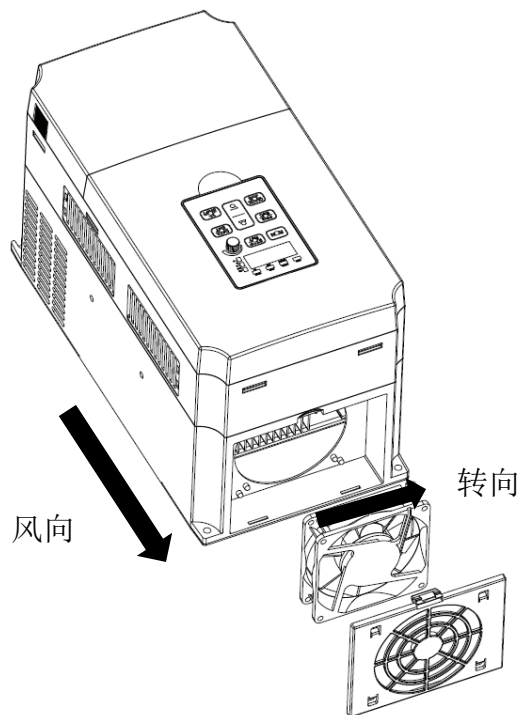
三相 380V 11-15KW 机器风扇维护示意图
