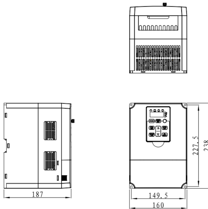
5.5KW-7.5KW 结构示意图及尺寸
