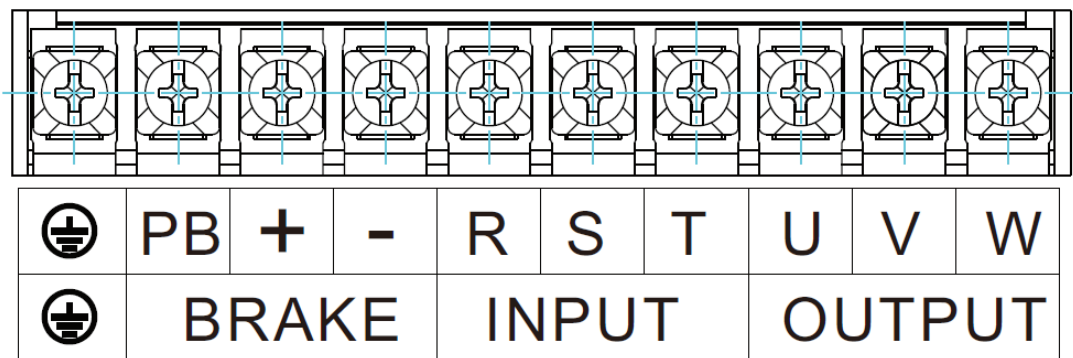
11KW-22KW 主回路端子示意图
