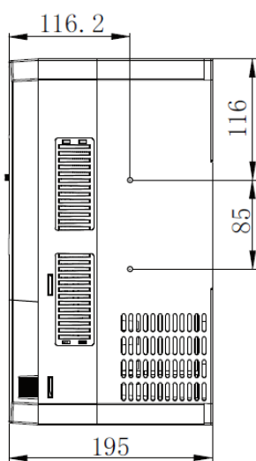
18.5KW—22KW 结构示意图及尺寸
