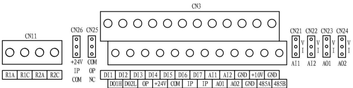
5.5KW-7.5KW 控制端子示意图
